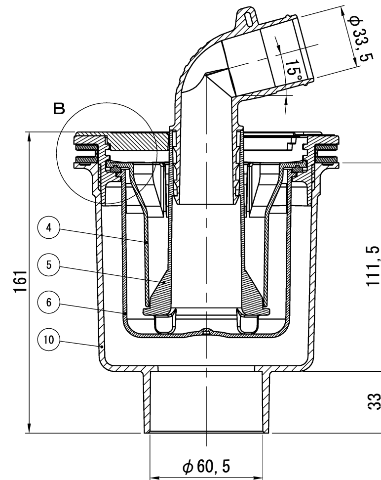
断面A-A
